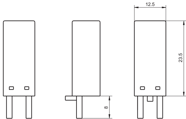
外形尺寸图
